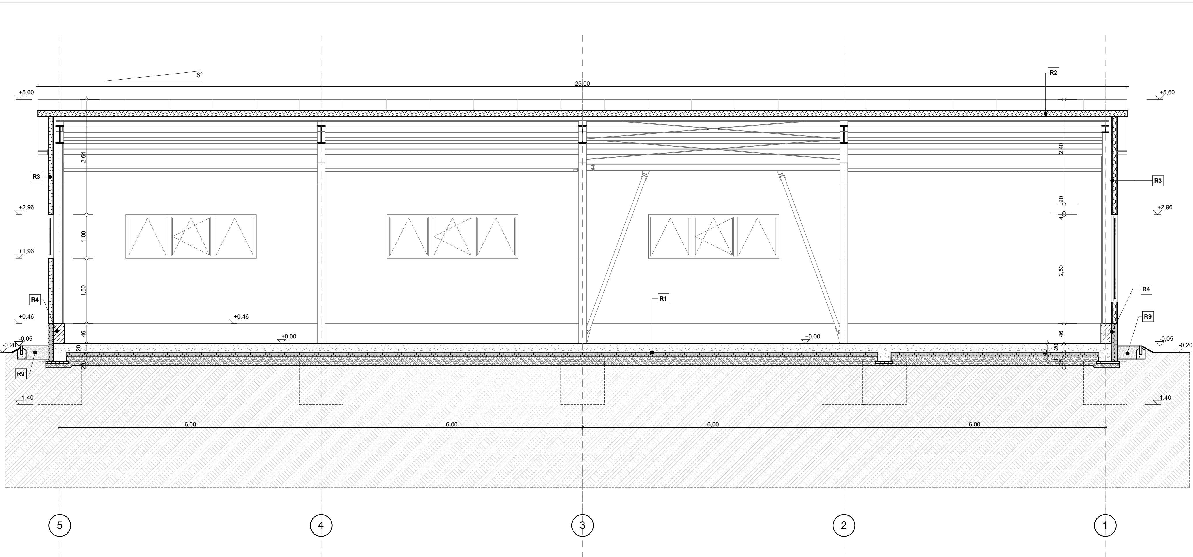
C-C METSZET M=1:100
