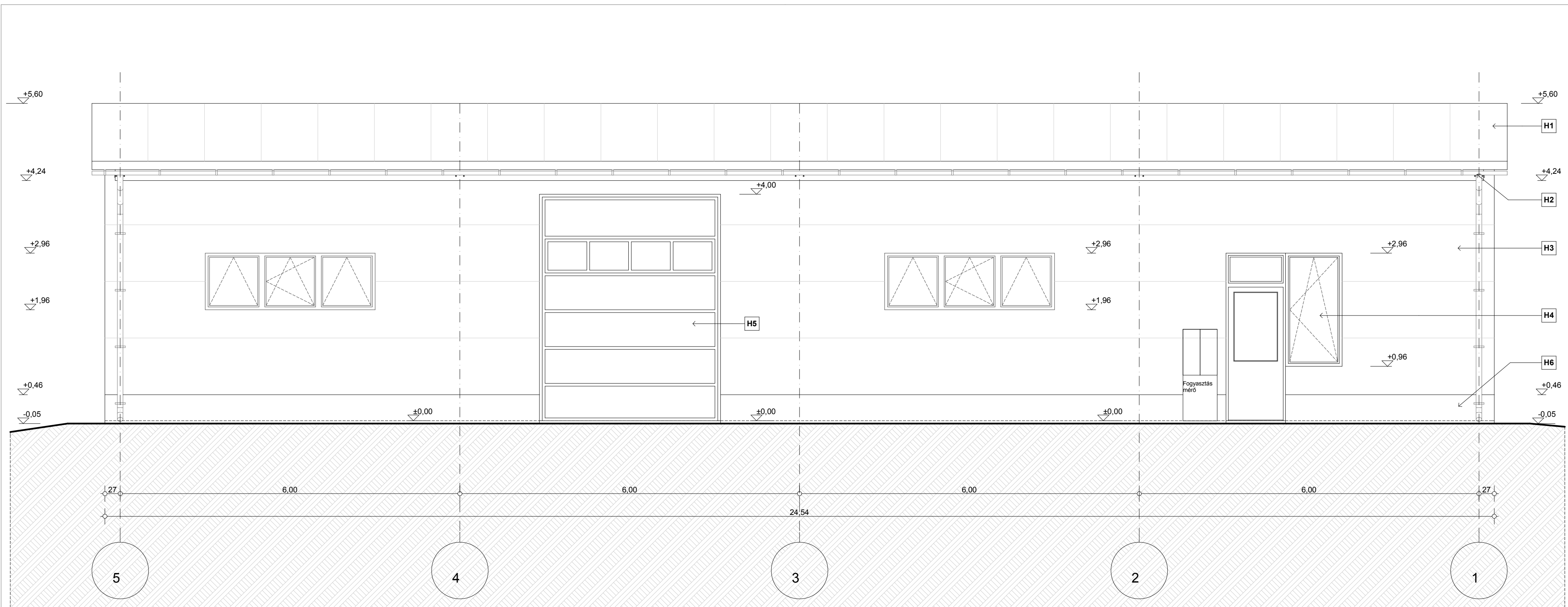
DÉLI HOMLOKZAT M=1:100
