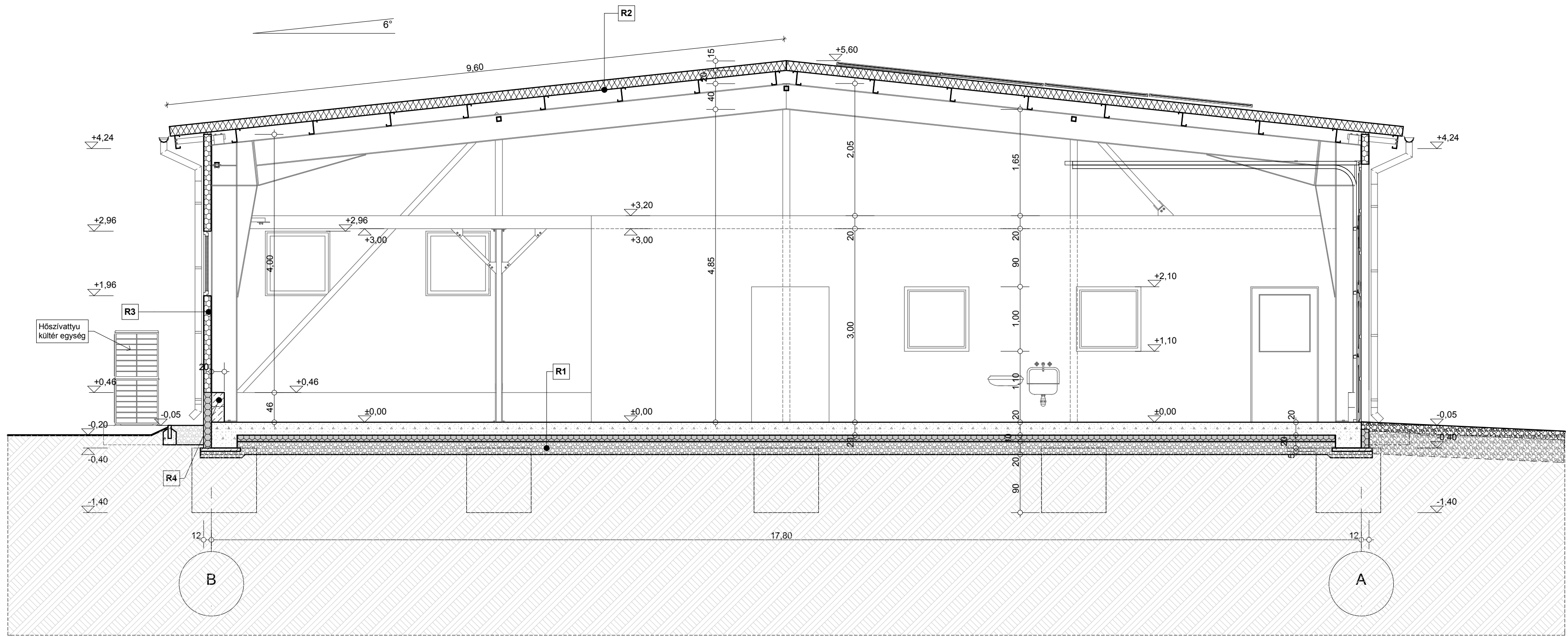
A-A METSZET M=1:50
