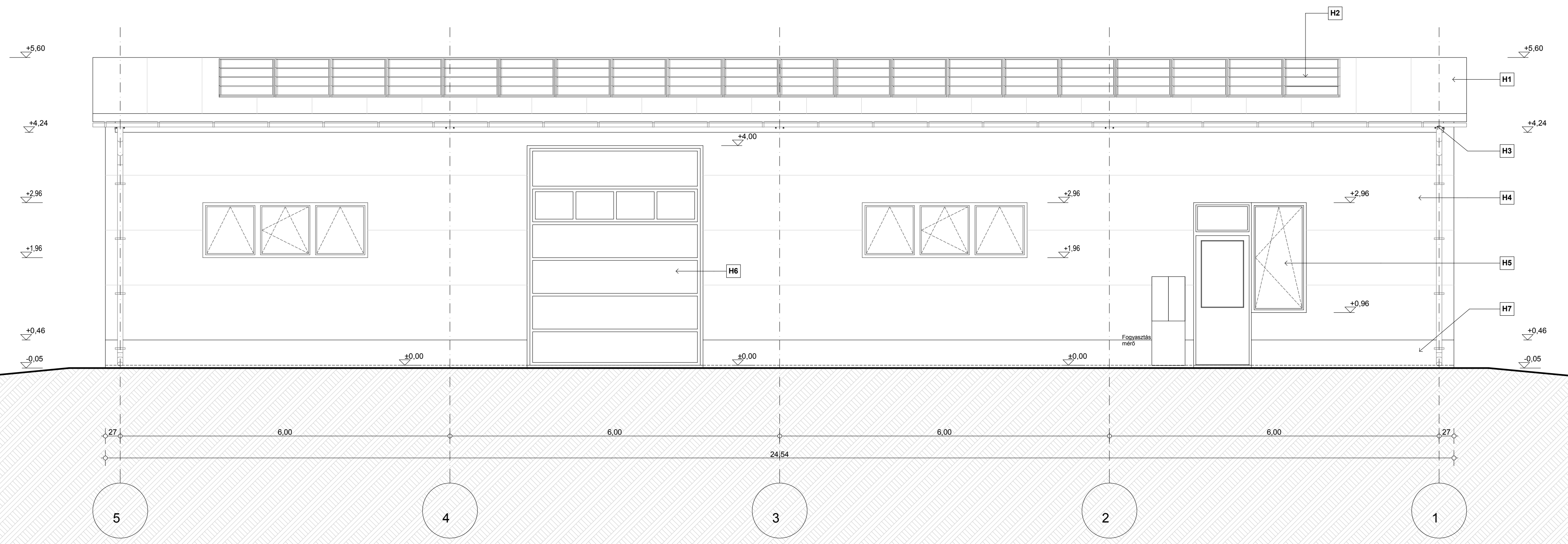
DÉLI HOMLOKZAT M=1:50
