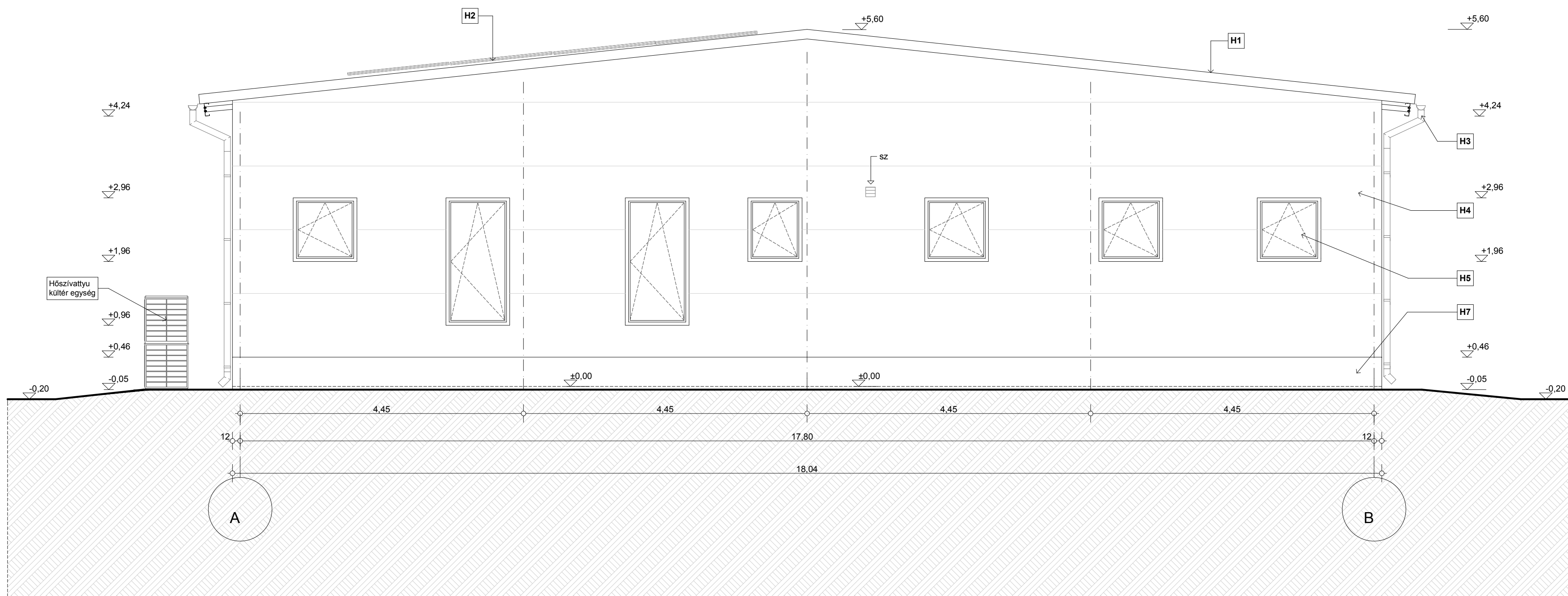
KELETI HOMLOKZAT M=1:50
