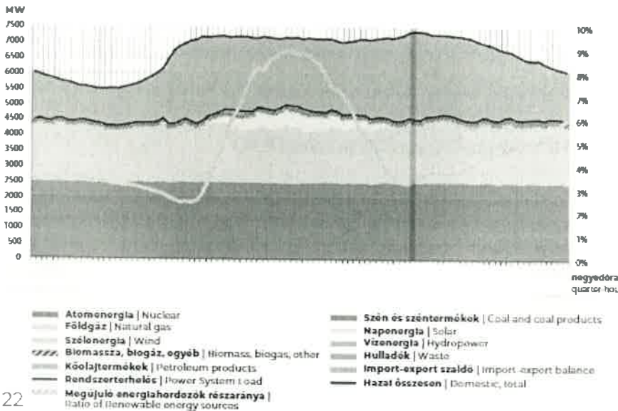
NAPI BRUTTÓ TERHELÉSI GÖRBE - ELSŐDLEGESEN HASZNÁLT ENERGIAHORDOZÓK SZERINT (TÉLI CSÚCS: 2022. JANUÁR 25. 17:00, 7 396 MW) DAILY GROSS SYSTEM LOAD PER PRODUCTION TYPE (WINTER PEAK LOAD: 25 JANUARY, 2022 17:00, 7 396 MW)
